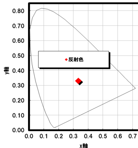
色彩特性:CIE1931 XYZ表色系 視野角10deg
