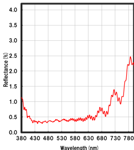
分光光度計による分光特性
