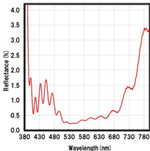
分光特性:HEA2000
