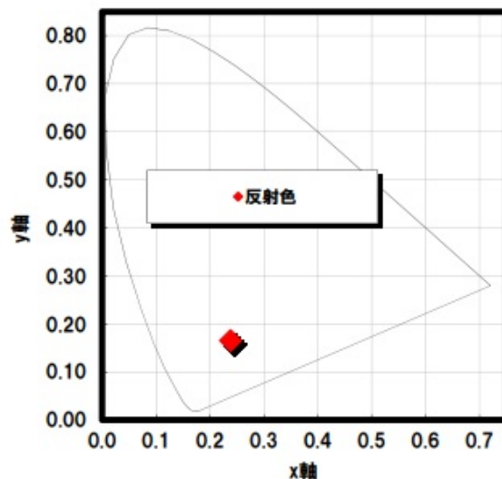
色彩特性:CIE1931 XYZ表色系 視野角10deg
